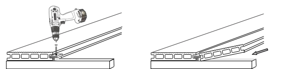
Prévisser et ne pas serrer complètement les clips afin de pouvoir insérer la deuxième lame en dessous
