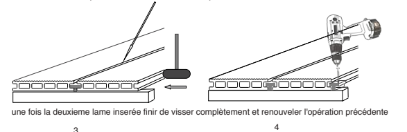
Espacement entre les lames à respecter
